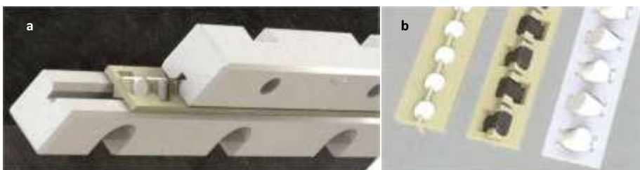
Rys. 5. Ceramiczne prowadnice liniowe: a) struktura konstrukcyjna w złożeniu, b) przykładowe elementy składowe [3]
