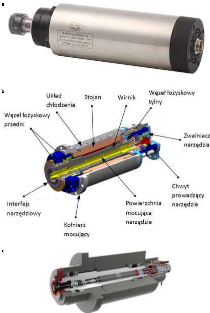
Rys. 4. Przykłady wrzecienników kompaktowych: a) widok (φ 80×200 mm, N=2,2 kW, n=400 s -1 ), b i c) przekroje
