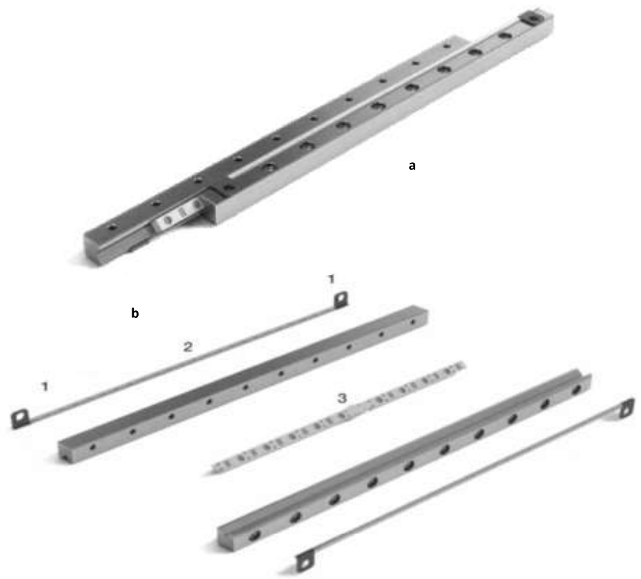
Rys. 7. Przewodnice liniowe z wymuszonym prowadzeniem koszyka: a) widok kompletnej przewodnicy, b) elementy składowe przewodnicy: 1 – zaciski listwy zębatej, 2 – listwy zębate, 3 – koszyk z kołami zębatymi [4]
